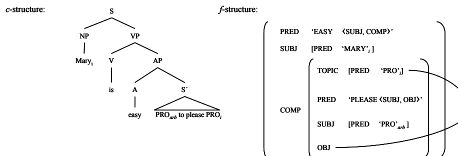
LFG repræsentationen af Mary is easy to please f-strukturen efter Dalrymple & King (2000:12)
